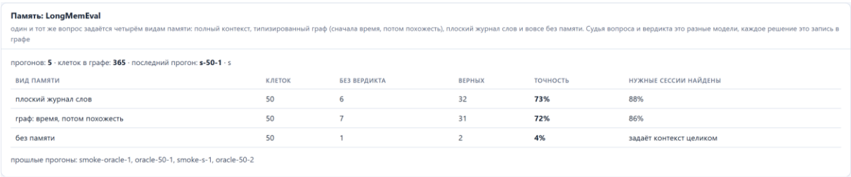
Рисунок Г.3. Раздел памяти: сравнение видов памяти на публичном наборе и честное состояние замера.
